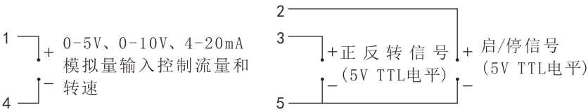
4-20mA、0-5V、0-10V外控输入模块接线图
